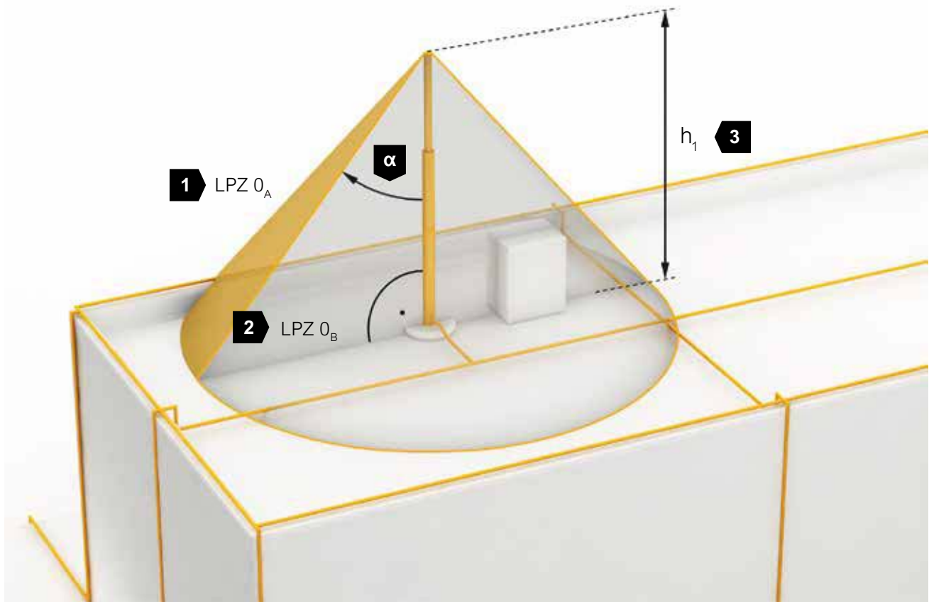
Рис. 2.10: Рассчитанная на основе упрощенного метода защитного угла защитная площадь молниеприемного стержня.
