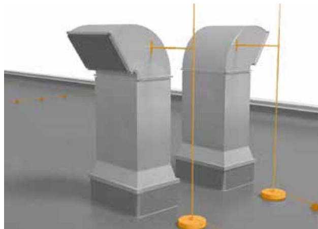
Рис. 2.31: Молниеприемный стержень с регулируемой изолированной траверсой
