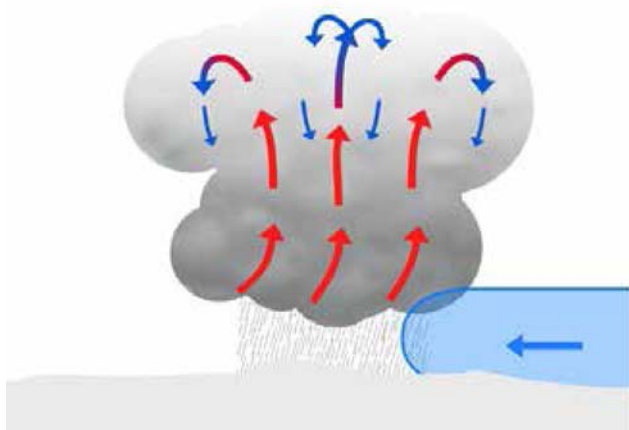
Рис. 1.3: Холодный воздушный фронт
